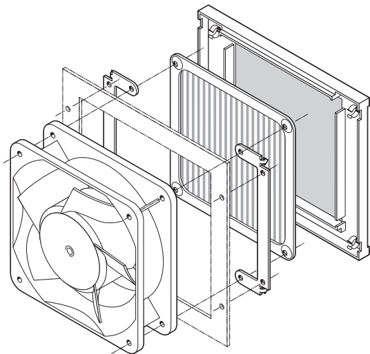
LZ60 Grobfilter
